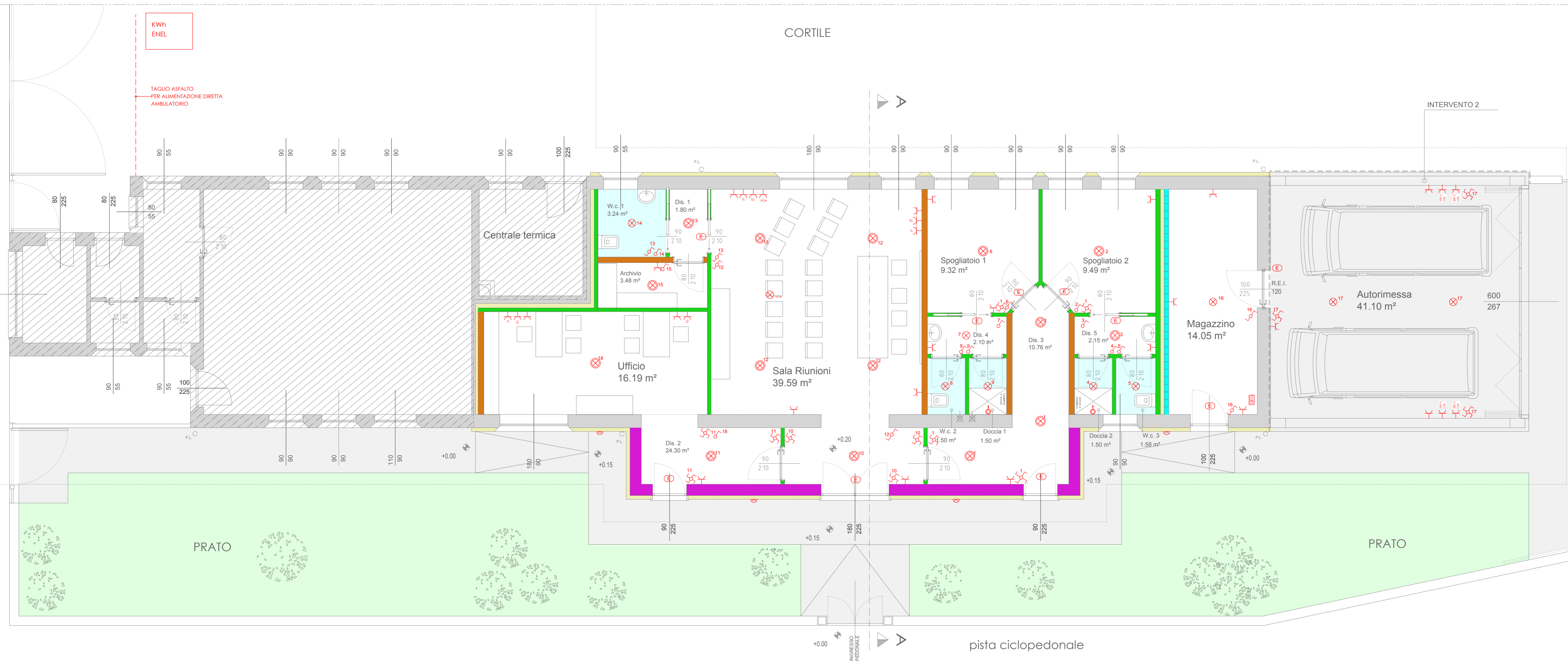
pianta piano terra : progetto scala 1:100
