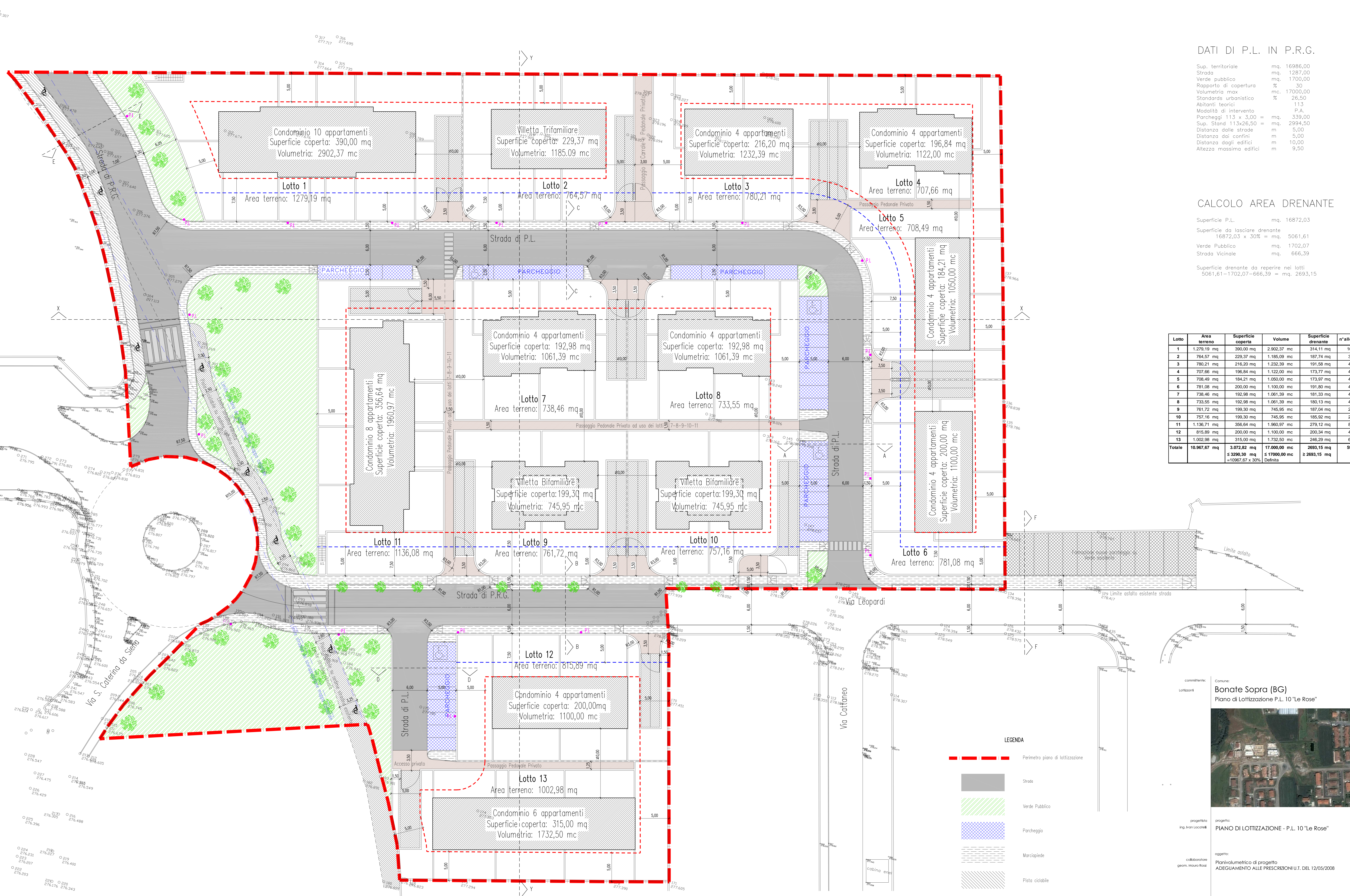
PLANIMETRIA scale 1:200
